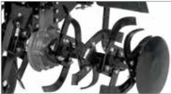
Transmisión de engranajes en baño de aceite, resistente y de bajo mantenimiento.
